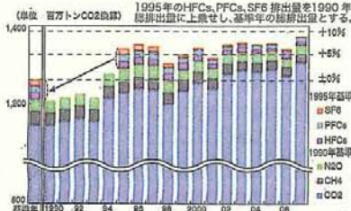
図 日本温室効果ガス排出量の推移 (1990-2007年) (単位: 百万トンCO2当量)
